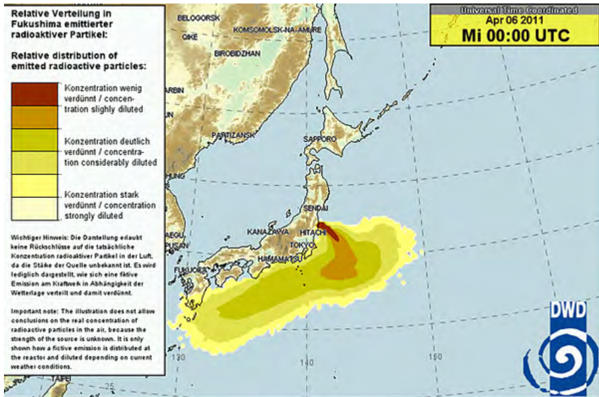
放射性物質の拡散予測(6日0時を想定) = ドイツ 気象局ホームページより(画像クリックで同サイトへ)
